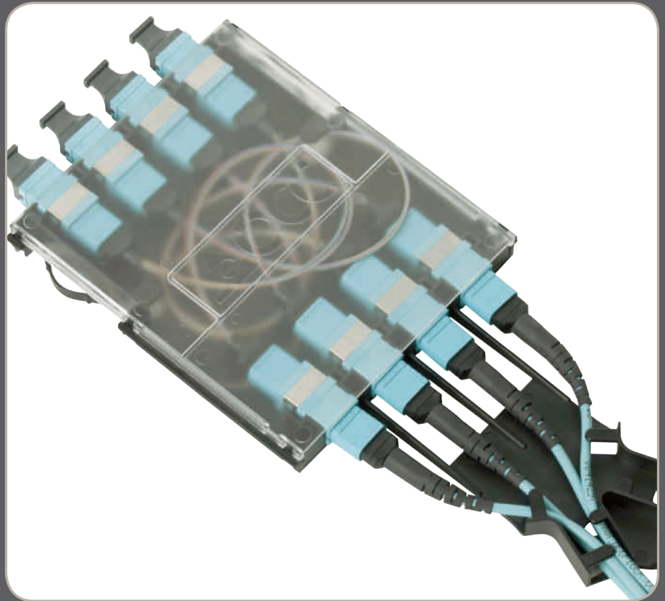
Procyon MTP-MTP Cassette
