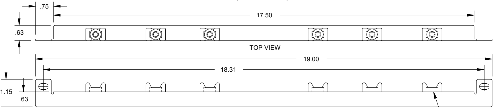
CABLE MGMT BAR (OCC P/N CMB19)
