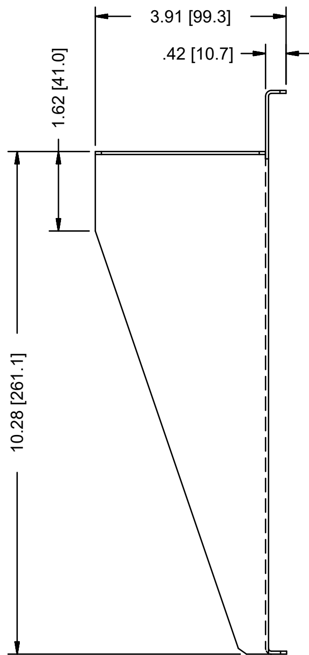
LEFT SIDE
