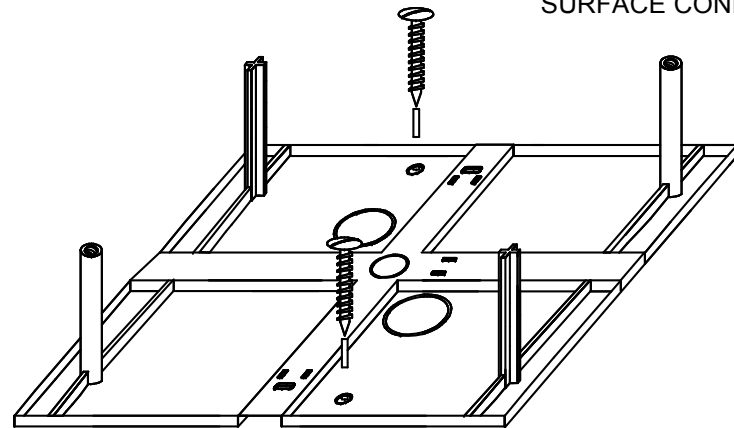
CUTOUTS TO FIT SURFACE CONDUIT
