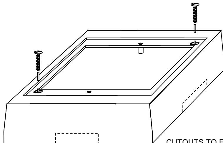
CUTOUTS TO FIT SURFACE CONDUIT
