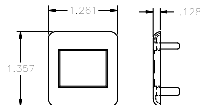
LC/SC BEZEL
