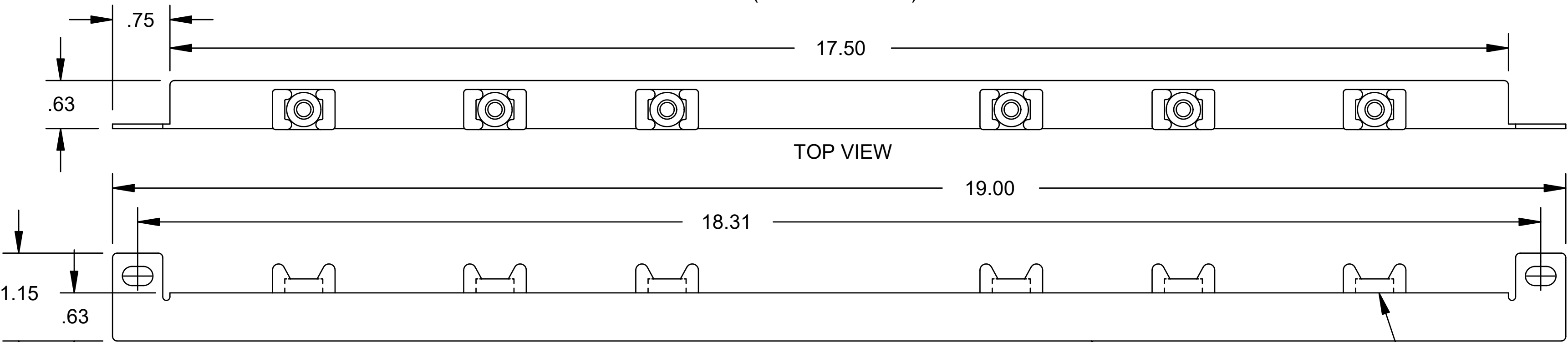
CABLE MGMT BAR (OCC P/N CMB19)
